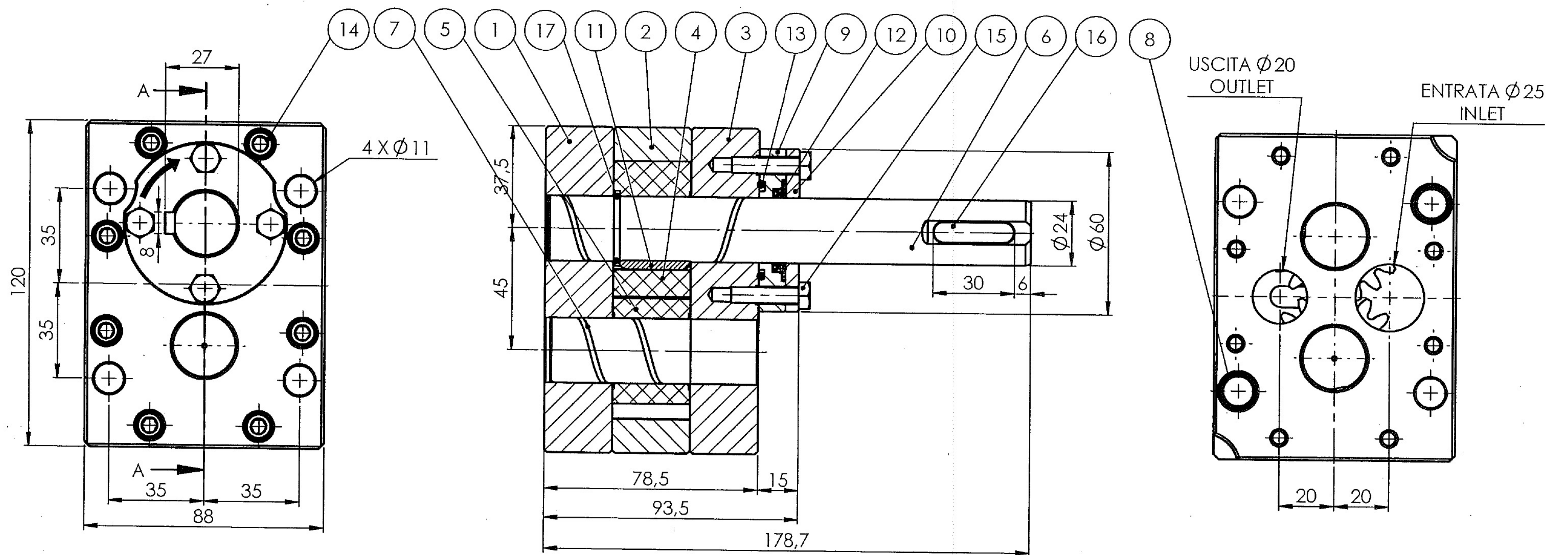
SEZIONE A-A
