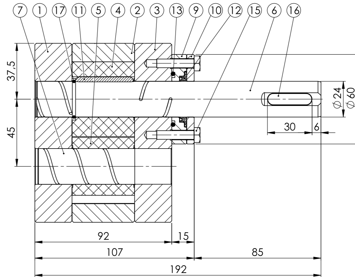
SEZIONE A-A
